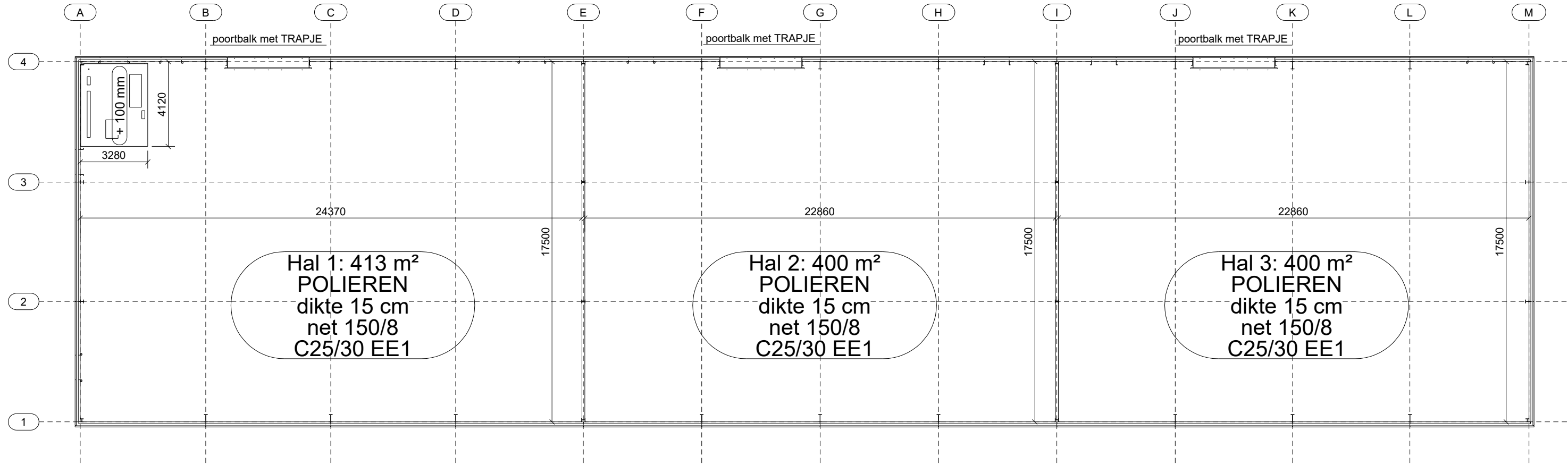
Grondplan
